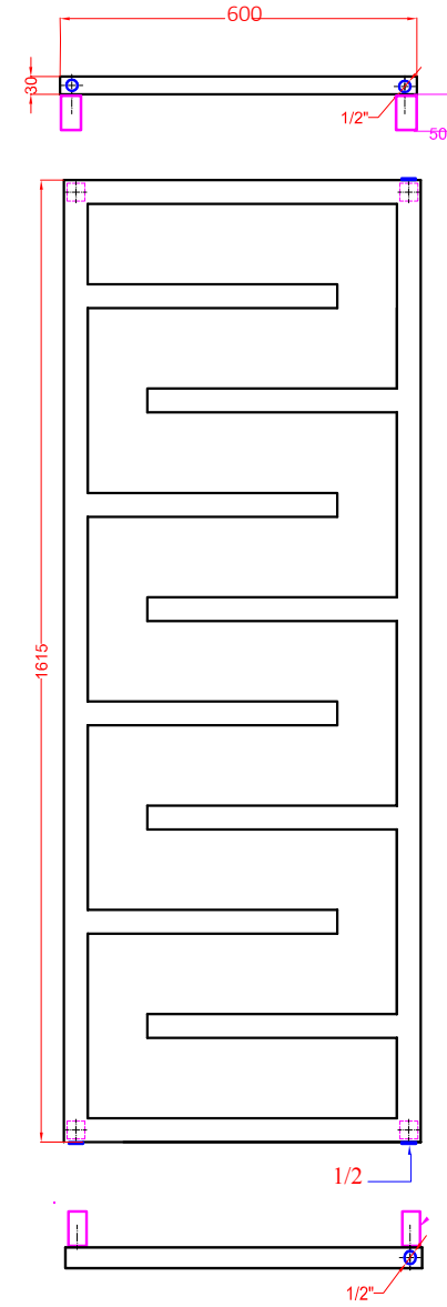
Pipe Centres= 560mm
