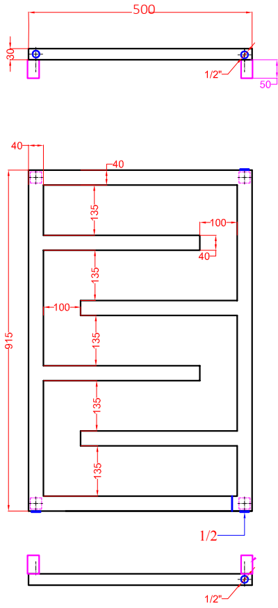
Pipe Centres= 460mm
