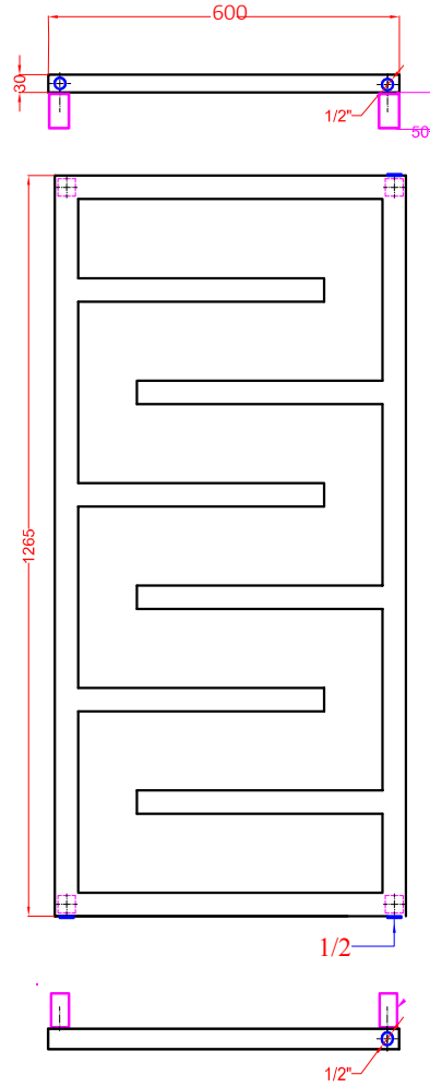
Pipe Centres= 560mm
